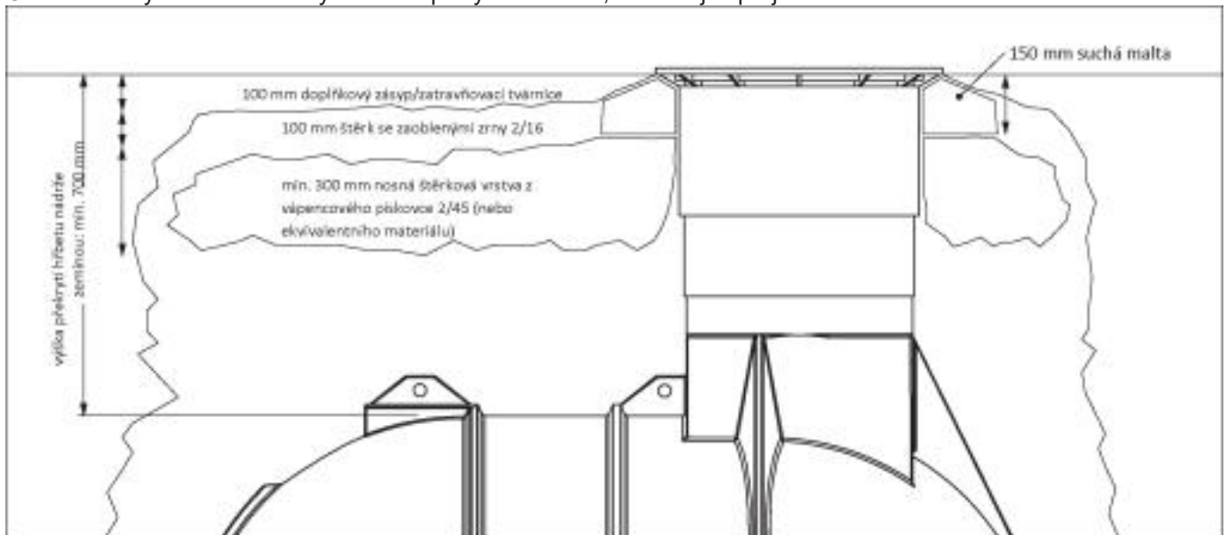
Obrázek 2: Vytvoření nástavby s teleskopickým tubusem, umožňující přejíždění osobních vozidel na daném místě
