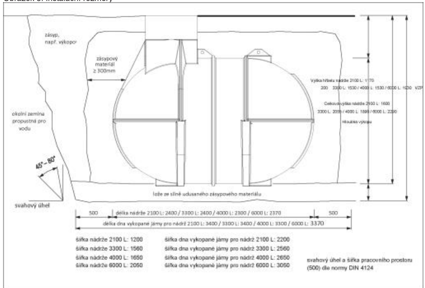
Obrázek 3: Instalační rozměry
